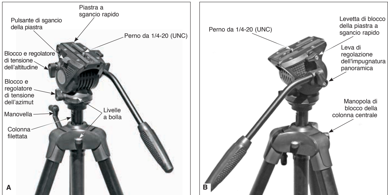
Figura 2. (A) Testa di panoramica Tritech II, lato sinistro e (B) lato destro.
