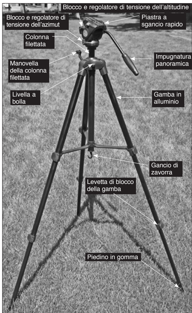
Figura 1. Treppiede da esterni Trittech II con gambe estese
